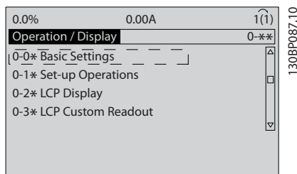
Рисунок 5.3 Управ./Отображ.
