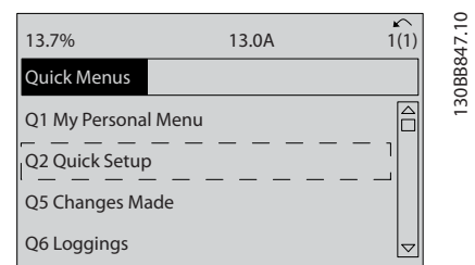
Рисунок 3.29 Быстрые меню
