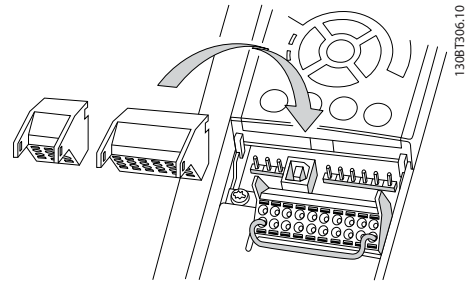
Рисунок 2.20 Удаление клемм управления
