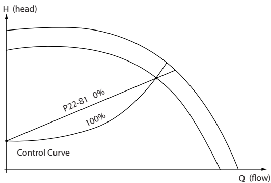
Рисунок 3.59 Квадратично-линейная аппроксимация характеристики
