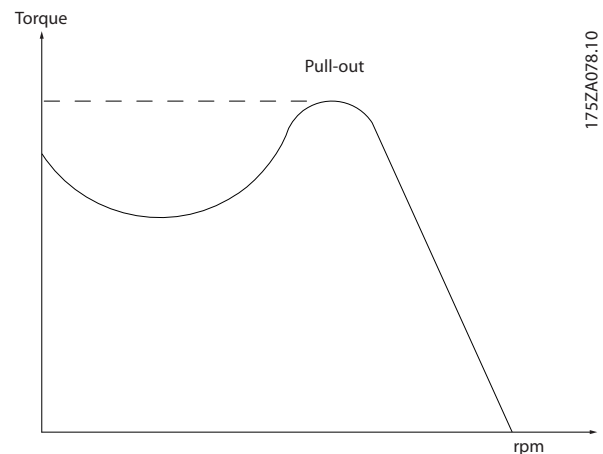
Рисунок 1.1 Момент опрокидывания
