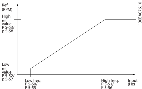
Рисунок 3.27 Импульсный вход
