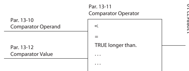
Рисунок 3.36 Компараторы
