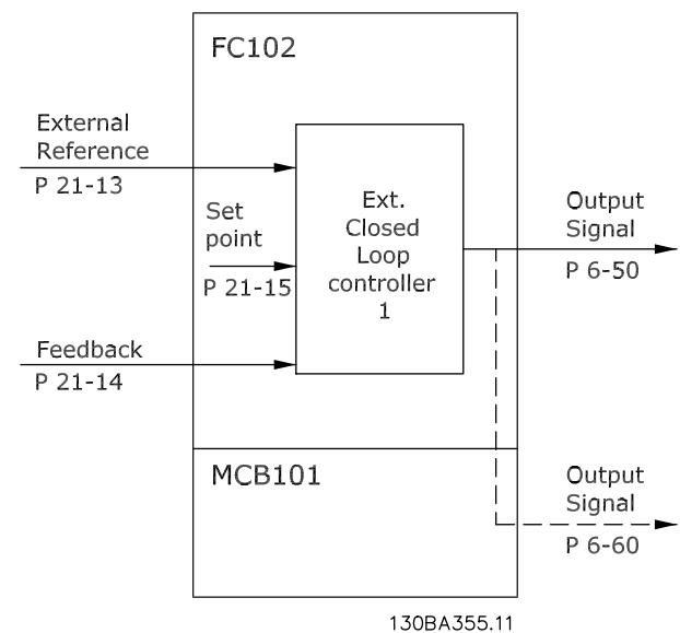
Рисунок 3.50 Расшир. CL 1, задан./обр.связь
