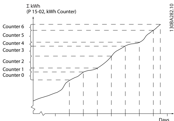
Рисунок 3.63 График энергопотребления
