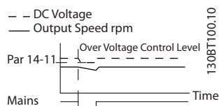
Рисунок 3.42 Кинетический резерв, короткое замыкание сети. Скачок происходит, пока в системе есть энергия.
