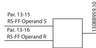
Рисунок 3.37 Триггеры сброса/установки
