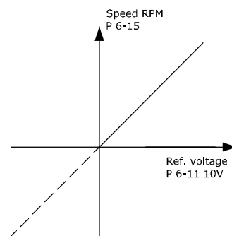
Рисунок 1.9 Задание от потенциометра
