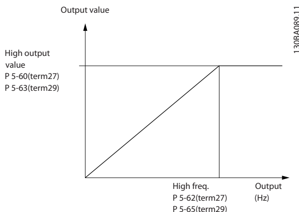
Рисунок 3.28 Импульсный выход
