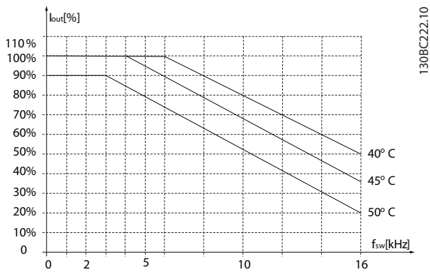
Рисунок 8.6 400 В, IP20, H3, 5,5–7,5 кВт
