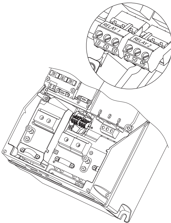
Рисунок 5.18 Габарит корпуса 16 IP54 380–480 В 22–37 кВт
