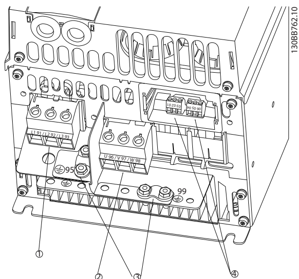
Рисунок 5.3 Габарит корпуса N6 IP20 380–480 В 30–45 кВт IP20 200–240 В 15–18,5 кВт IP20 525–600 В 22–30 кВт
