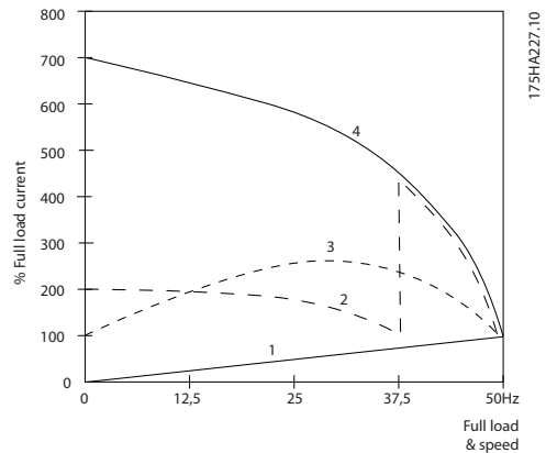
Рисунок 2.8 Пусковой ток
