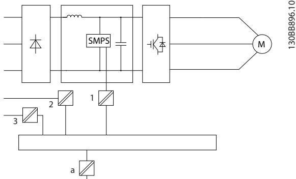
Рисунок 2.25 Гальваническая развязка
