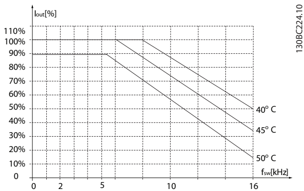
Рисунок 8.8 400 В, IP20, H4, 11–15 кВт
