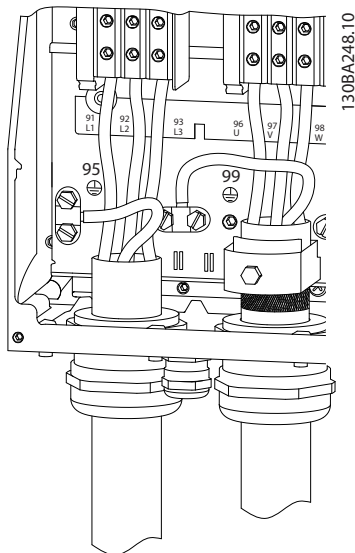
Рисунок 5.19 Габарит корпуса 17, 18 IP54 380–480 В 45–55 кВт IP54 380–480 В 75–90 кВт
