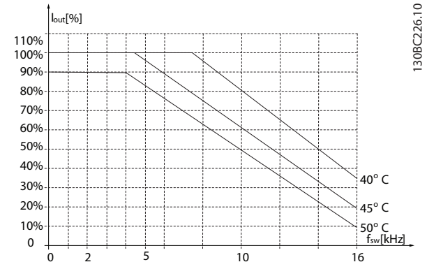
Рисунок 8.10 400 В, IP20, H5, 18,5–22 кВт
