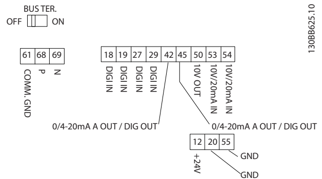
Рисунок 5.24 Клеммы управления
