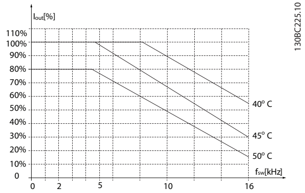
Рисунок 8.9 200 В, IP20, H5, 11 кВт
