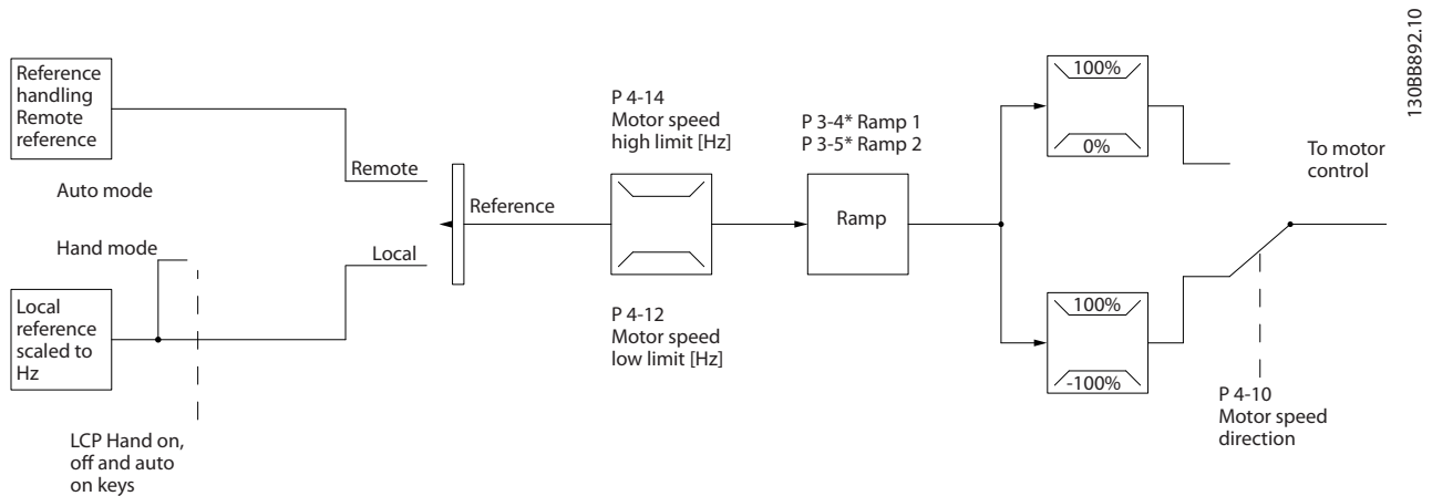
Рисунок 2.17 Структура разомкнутого контура
