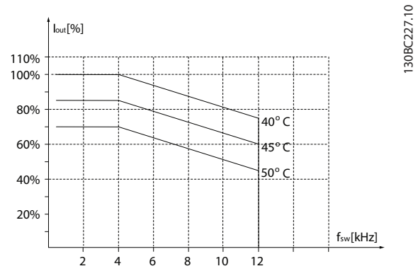
Рисунок 8.11 200 В, IP20, H6, 15–18,5 кВт
