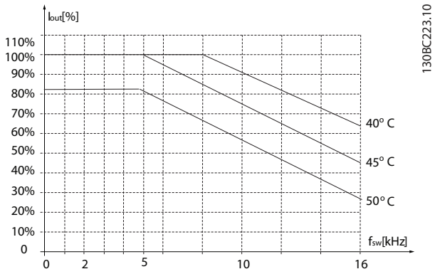
Рисунок 8.7 200 В, IP20, H4, 5,5–7,5 кВт
