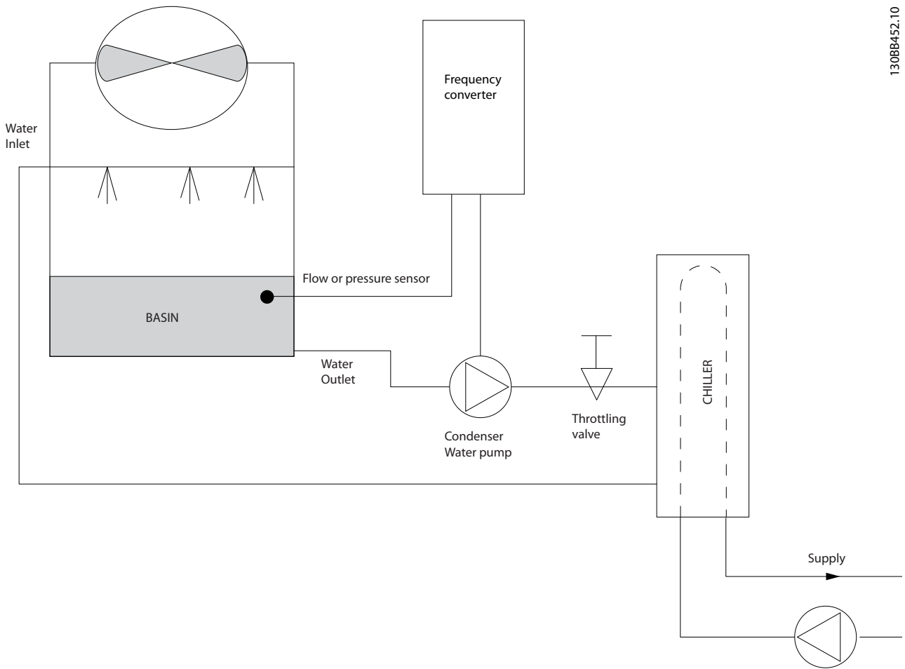
Рисунок 2.14 Использование преобразователя частоты с насосом конденсатора
