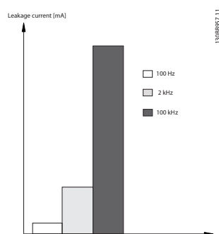
Рисунок 2.32 Влияние частоты RCD
