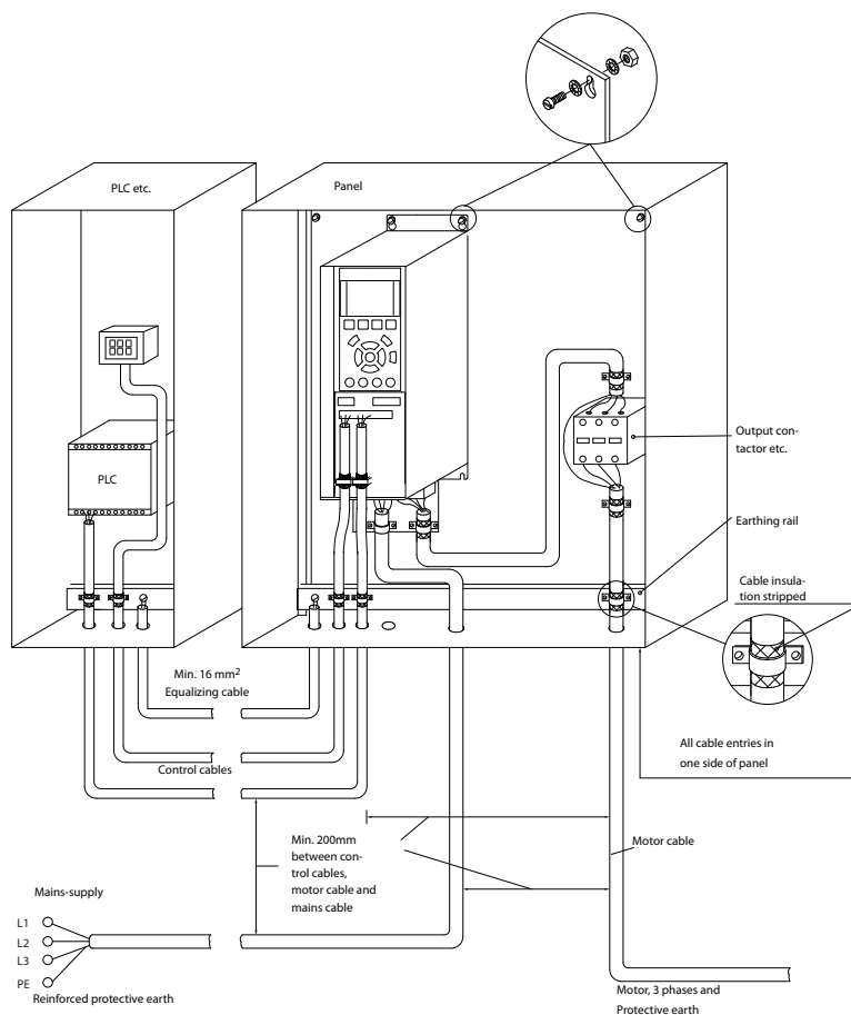
Рисунок 5.103 Корректный с точки зрения ЭМС электрический монтаж преобразователя частоты в шкафу
