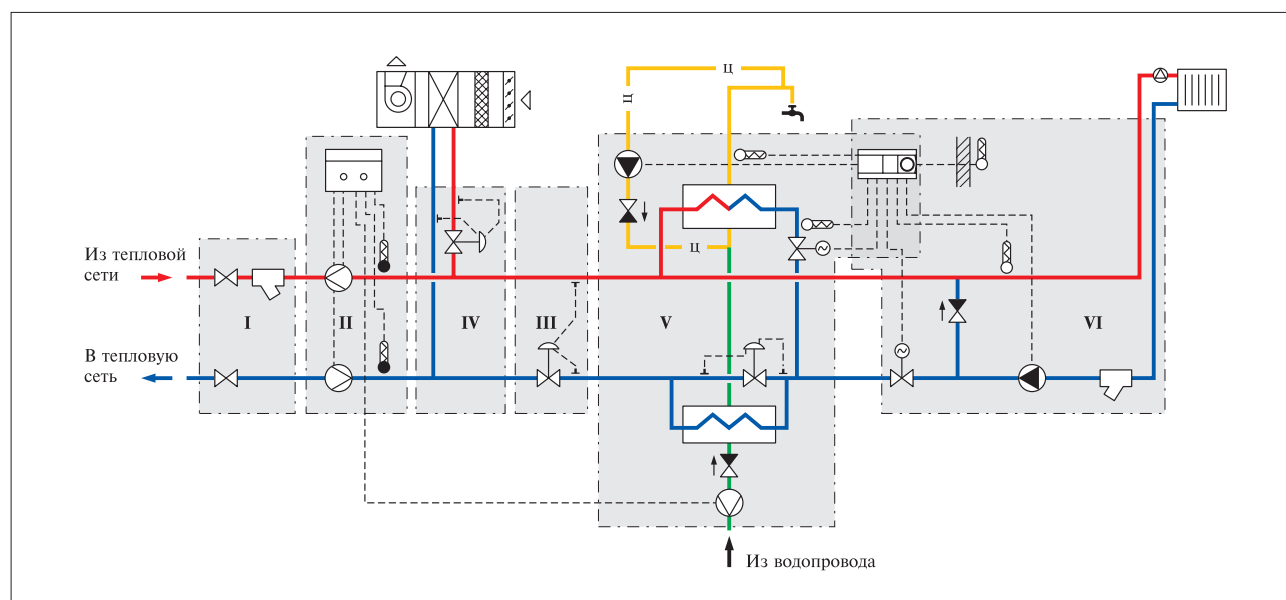
Рис. 3. Пример технологической схемы автоматизированного теплового пункта при закрытой системе теплоснабжения и зависимом присоединении системы отопления к тепловой сети.
