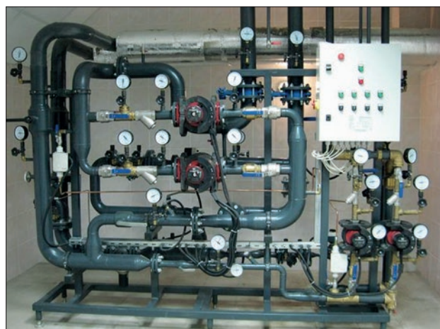
Рис. 2. Пример теплового пункта блочного исполнения с оборудованием, приборами и устройствами Danfoss.
