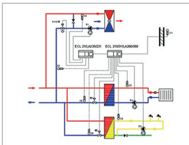
Рис. 53. Принципиальная схема автоматизации теплового пункта: система отопления, ГВС и calorifer системы вентиляции.
