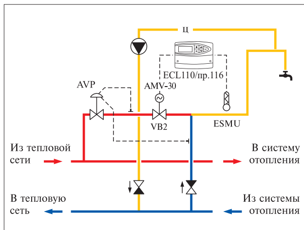
Рис. 8. Узел смешения для ГВС при открытой системе теплоснабжения.
