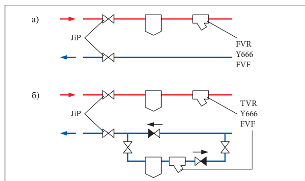
Рис. 5. Узел ввода. а – традиционный, б – с реверсивным байпасом.
