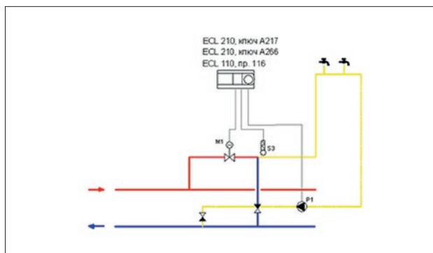
Рис. 49. Принципиальная схема автоматизации теплового пункта: ГВС при открытой системе теплоснабжения.
