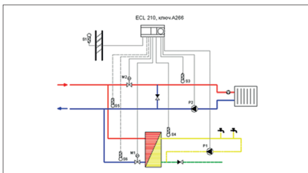
Рис. 51. Принципиальная схема автоматизации теплового пункта: система отопления и ГВС.
