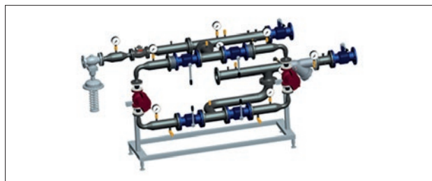
Рис. 41. Узлы смешения со 100% резервированием насосов (тип АУУ).
