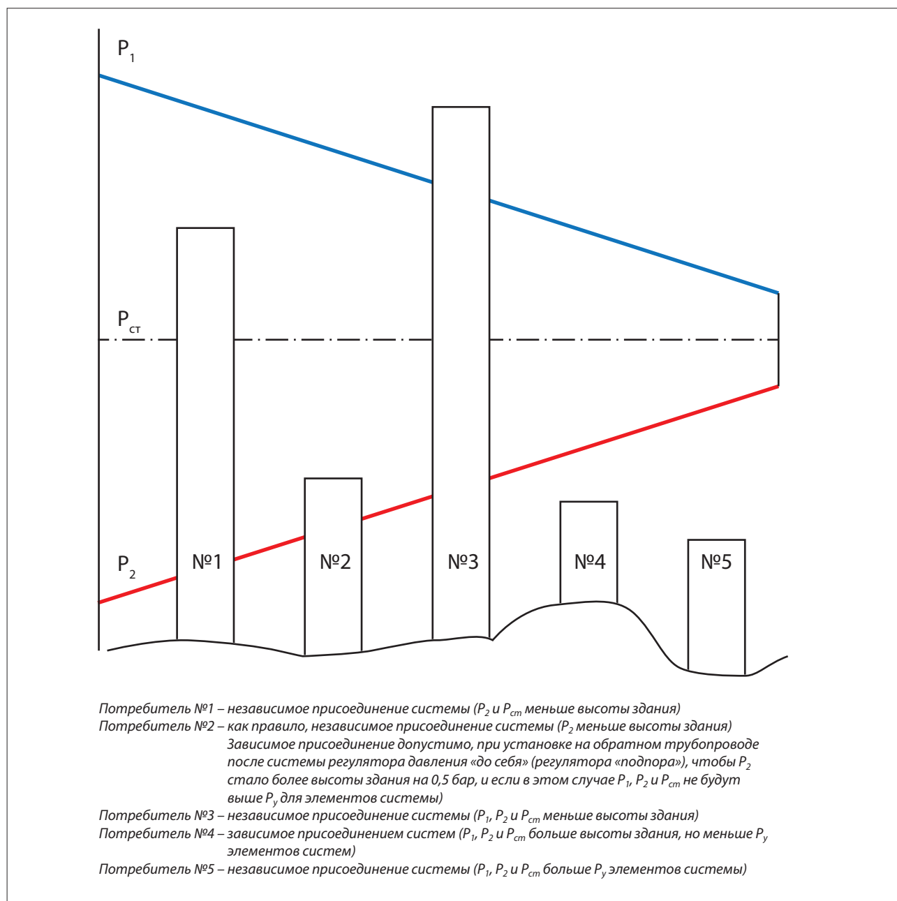
Рис. 7. Выбор способа присоединения систем отопления и вентиляции к тепловой сети.
