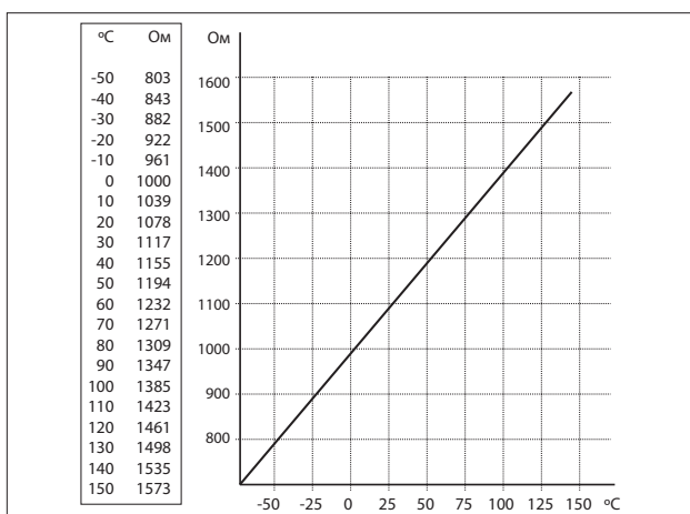
Рис. 23. Зависимость сопротивления датчиков Pt1000 от температуры.
