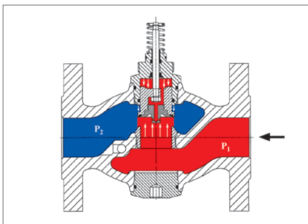
Рис. 31. Поршневая система разгрузки регулирующего клапана.
