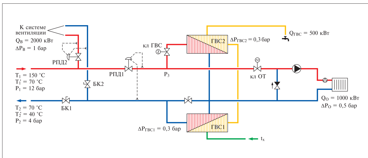
Рис. 56. Схема теплового пункта (к примеру 3).
