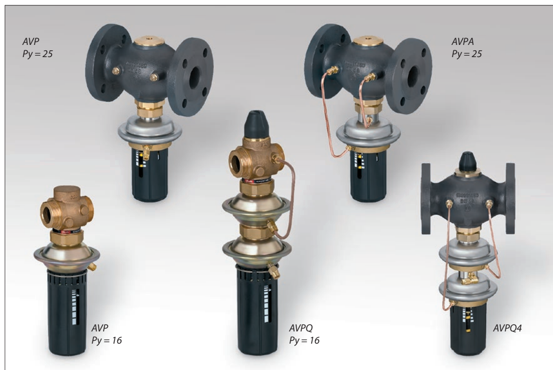
Рис. 32. Моноблочные регуляторы давления.
