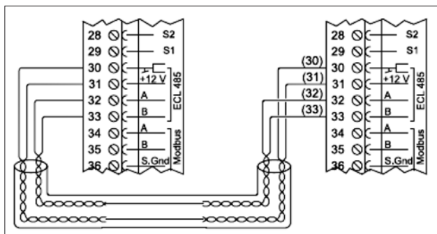
Рис. 19. Схема объединения двух контроллеров ECL Comfort 210/310 в локальную сеть.
