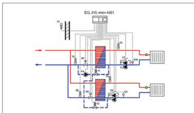
Рис. 48. Принципиальная схема автоматизации теплового пункта: два контура системы отопления с управляемой подпиткой.
