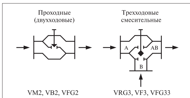
Рис. 29. Регулирующие клапаны с электроприводами.
