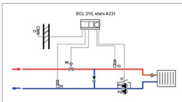
Рис. 45. Принципиальная схема автоматизации теплового пункта: система отопления при зависимом присоединении к тепловой сети.
