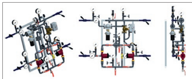
Рис. 40. Узлы смешения со 100% резервированием насосов (тип DH-RR).
