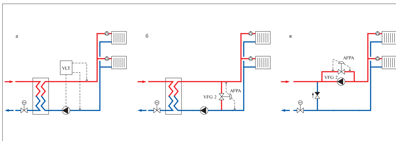
Рис. 9. Поддержание постоянного перепада давлений на двухтрубной системе отопления.
