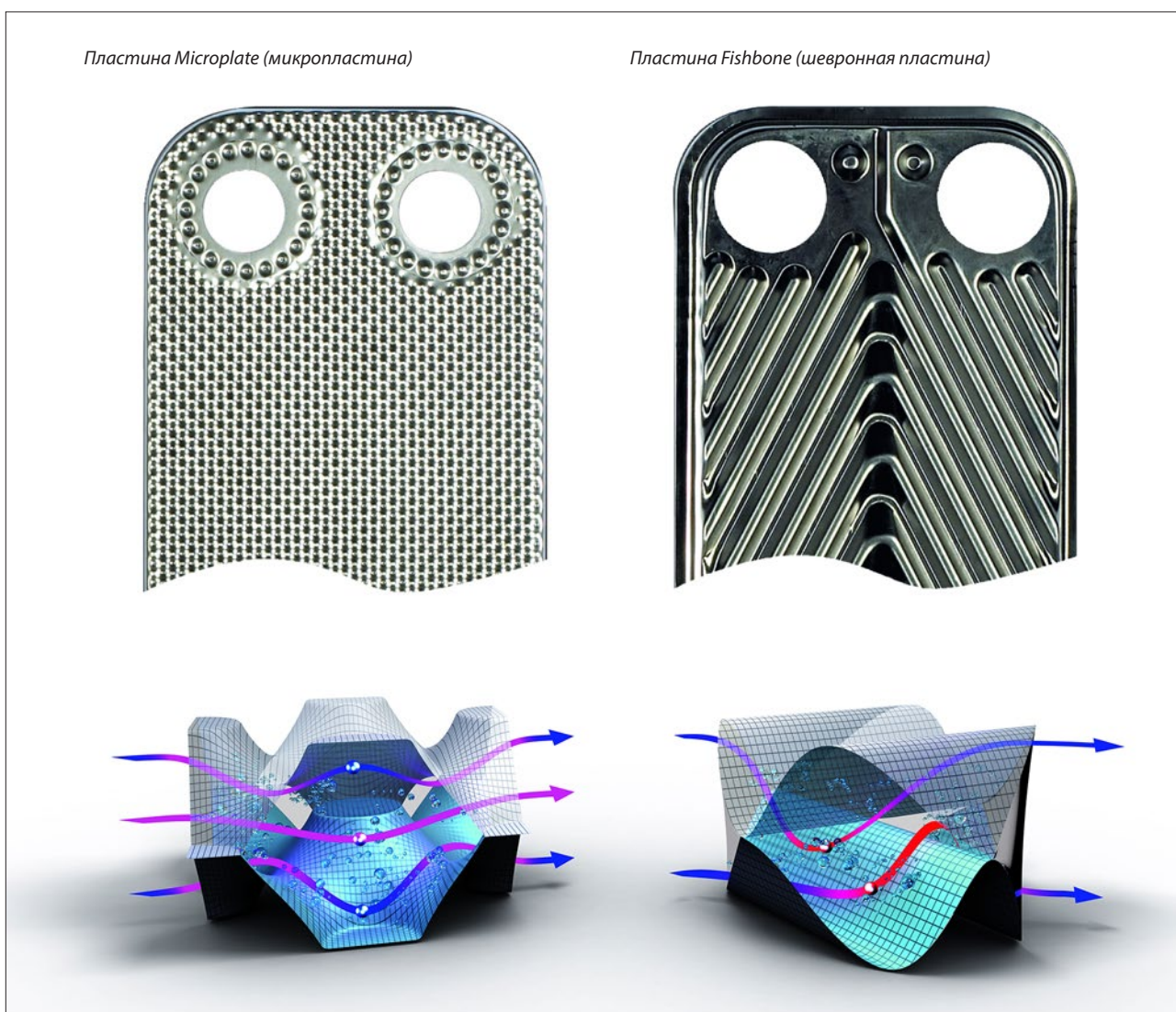
Рис. 34. Движение потока теплоносителя в микроканальных и шевронных теплообменниках
