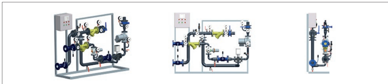
Рис. 39. Узлы смешения с одним насосом (одинарным или сдвоенным) тип US.
