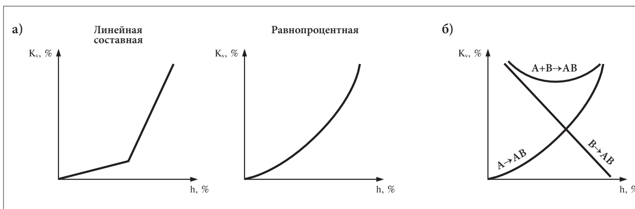
Рис. 30. Расходные характеристики: а) – проходных клапанов, б) – трехходовых клапанов.
