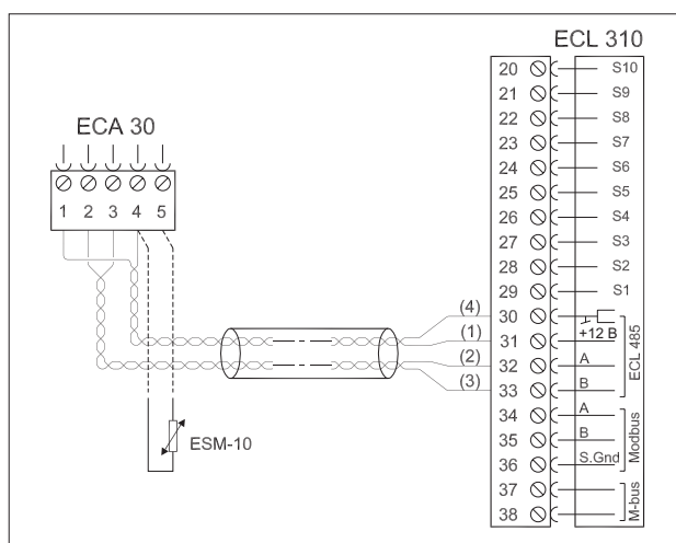
Рис. 17. Схема подключения блока дистанционного управления ECA 30 к регуляторам ECL Comfort 210/310.
