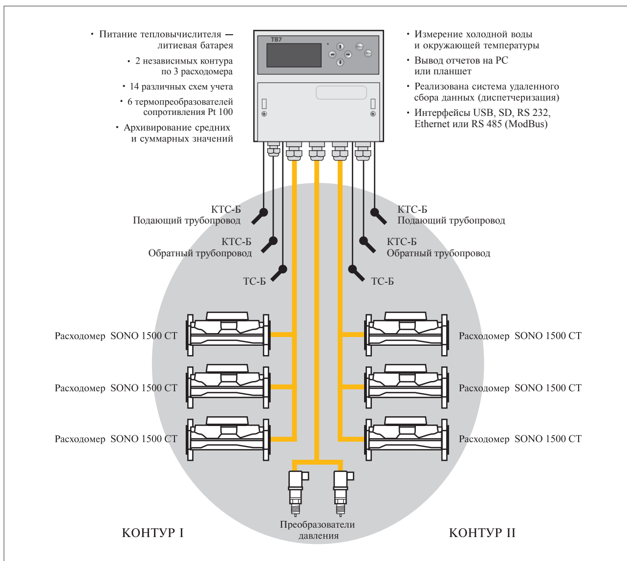
Рис. 6. Схема комплектации теплосчетчика T-34.
