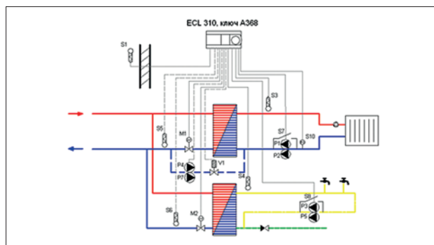
Рис. 52. Принципиальная схема автоматизации теплового пункта: система отопления с управлением подпиткой и ГВС.
