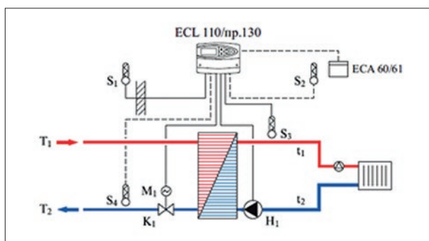
Рис. 44. Принципиальная схема автоматизации теплового пункта: система отопления при независимом присоединении к тепловой сети.
