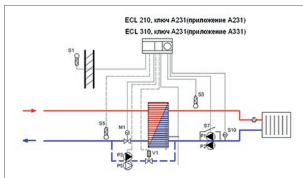
Рис. 46. Принципиальная схема автоматизации теплового пункта: система отопления с управляемой подпиткой.
