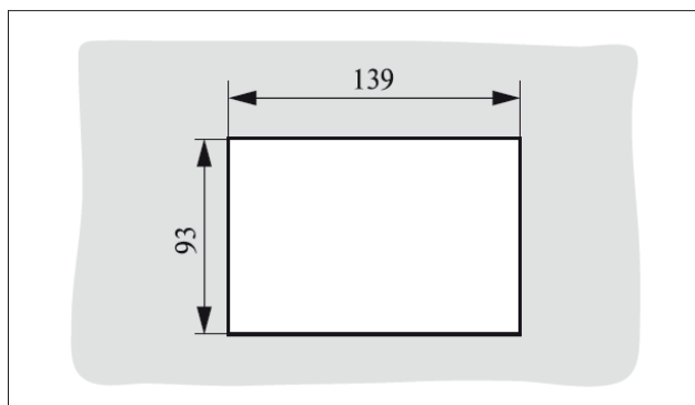
Рис. 13. Размеры отверстия в панели щита управления для установки ECL Comfort 110.
