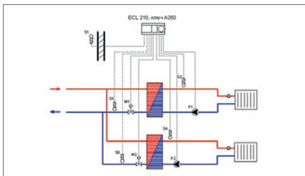
Рис. 47. Принципиальная схема автоматизации теплового пункта: два контура системы отопления.
