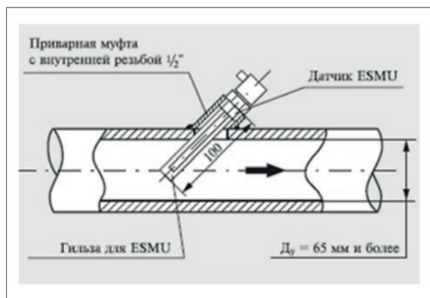
Рис. 27. Установка погружного датчика температуры ESMU.
