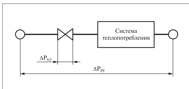
Рис. 55. Выбор перепада давлений на регулирующем клапане.
