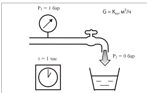
Рис. 54. Определение условной пропускной способности клапана.
