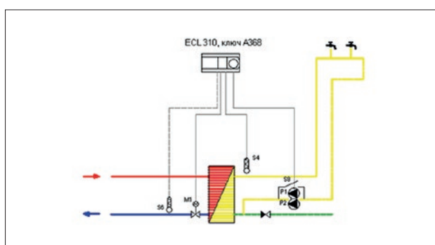
Рис. 50. Принципиальная схема автоматизации теплового пункта: ГВС при закрытом водоразборе.
