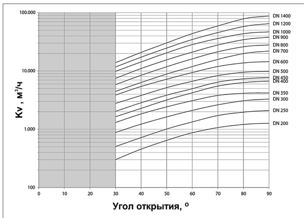
Диаграмма зависимости пропускной способности от угла открытия затвора
