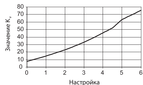
Расходная характеристика
