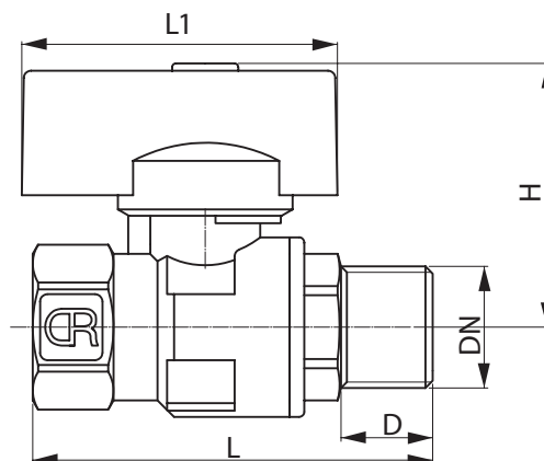
Сливной кран
