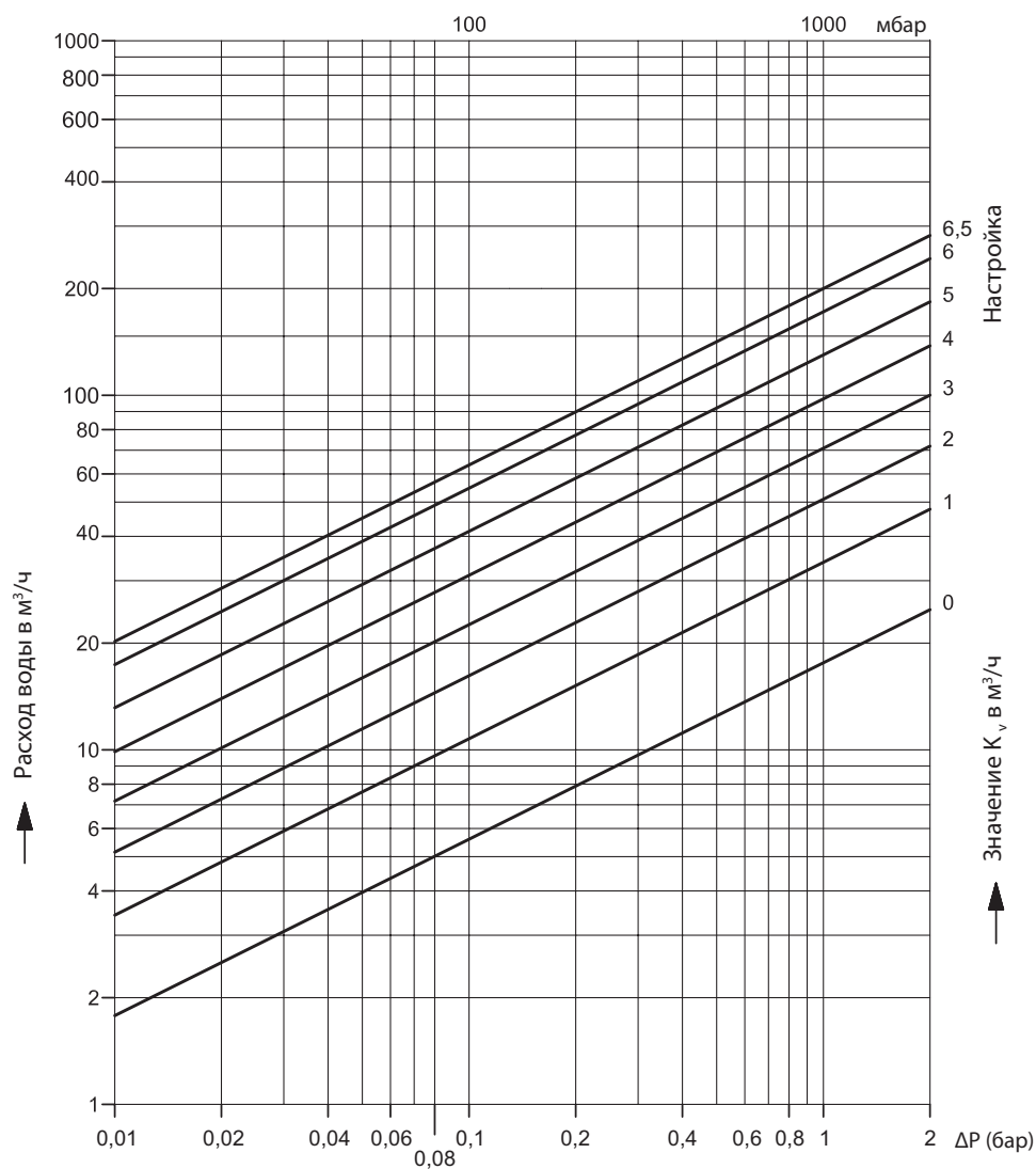
Расходная характеристика
